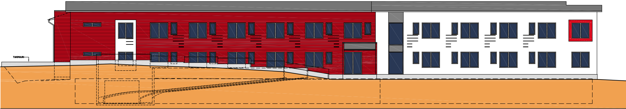
JULKISIVU ITÄÄN
